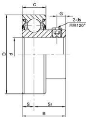
CSB200 带顶丝外圆柱面球轴承
