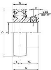
SB200 带顶丝外球面球轴承
