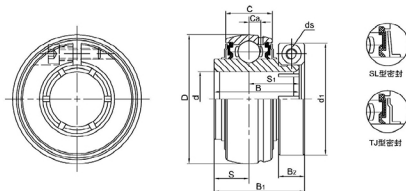
带同心套外球面球轴承
