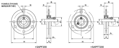
SAPFT200 SAPFT200 系列
