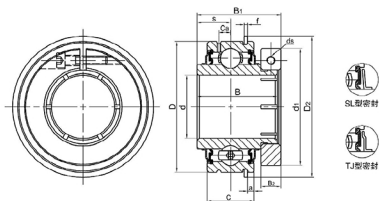
带止动环不锈钢球轴承
