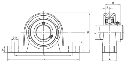
SSKP000 系列 立式带座 顶丝锁紧
