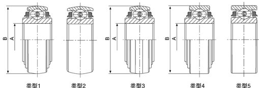
三唇密封非再调滑型农用轴承
