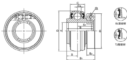
带同心套不锈钢外球面球轴承
