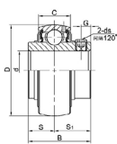
UC200 帶頂絲外球面球軸承
