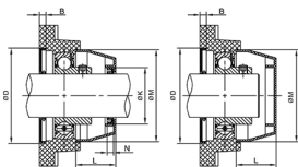
• 法兰带座
