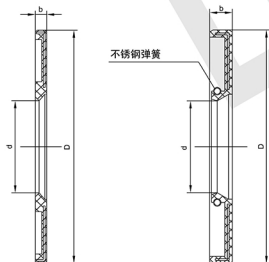
后油封
