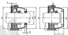
• 立式带座
