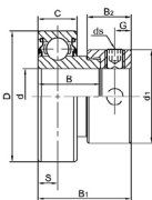
CSA200 带偏心套外圆柱面球轴承
