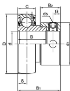
SA200(轻系列) 带偏心套外球面球轴承
