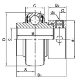
NA2000(HC200 UEL200) 带偏心套外球面球轴承
