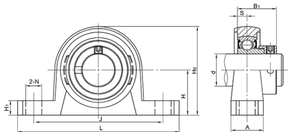
SSUP000 系列 立式带座 偏心套锁紧
