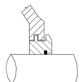
TSU 密封
