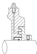
LS 端盖密封
