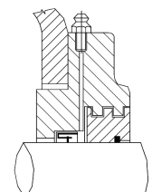
TAC 端盖密封
