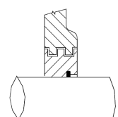
TS 密封
