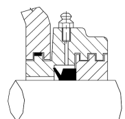
TST 端盖密封
