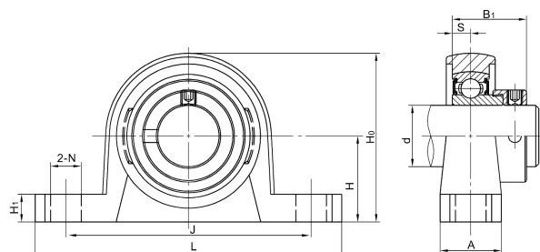
SSUP000 系列 立式带座 偏心套锁紧
