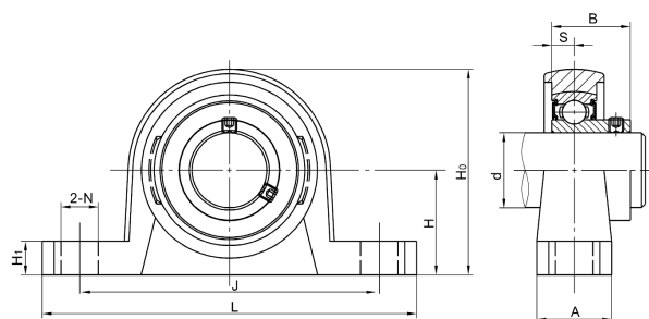
SSKP000 系列 立式带座 顶丝锁紧
