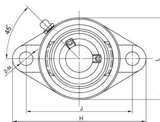
• SSUCFL200ESB (实心底)
