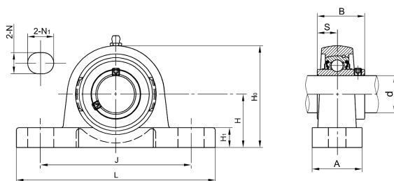
SSUCP200YHB (空心底)
