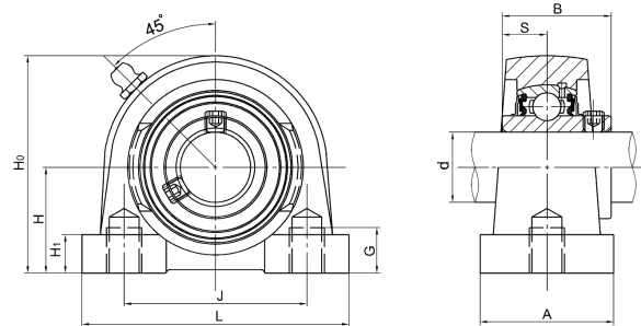
SSUCPA200 系列
