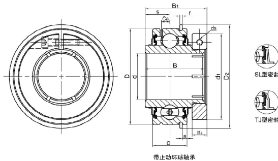
带止动环球轴承
