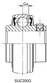
带顶丝不锈钢外球面球轴承
