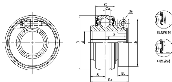
带同心套不锈钢外球面球轴承
