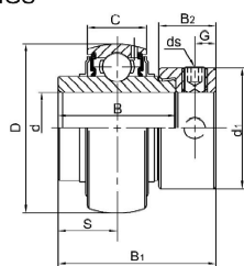
NA300(HC300 UEL300) 带偏心套外球面球轴承
