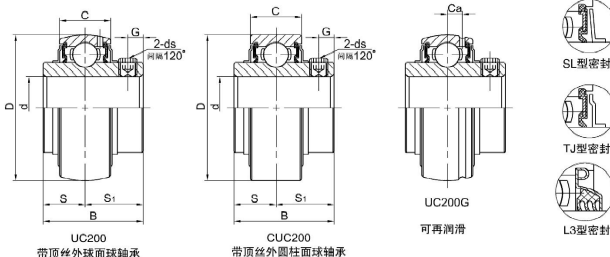
UC200 带顶丝外球面球轴承
