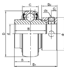
NA200(HC200 UEL200) 带偏心套外球面球轴承
