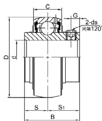
UCX00 带顶丝外球面球轴承
