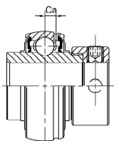
NA300G (重系列) 可再润滑型
