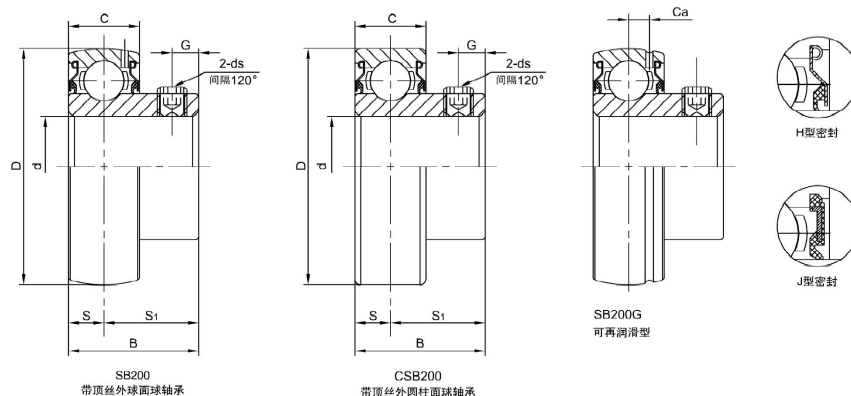
SB200 CSB200 系列
