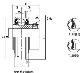
带止动环轴承
