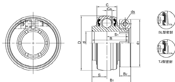
带同心套外球面球轴承
