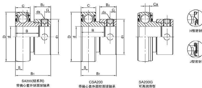
SA200 CSA200 系列
